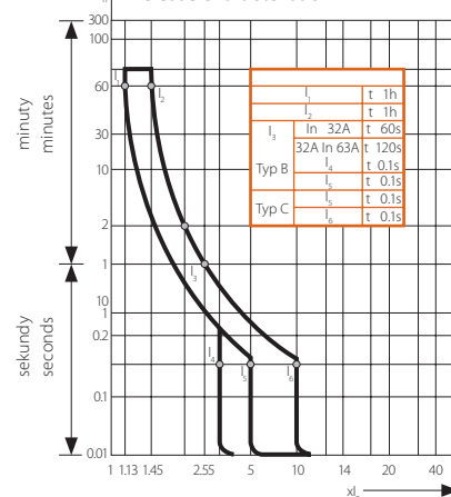
Charakterystyka wyzwalania Release characteristic
