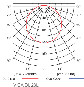
krzywa rozsyłu światłości / curve of intensity distribution η = 43%
