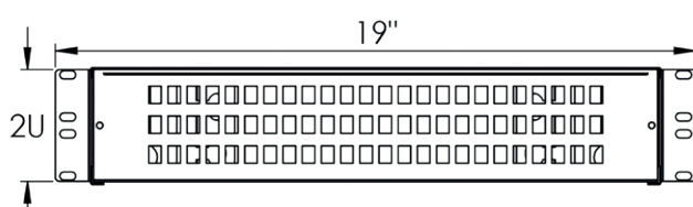
WIDOK PRZODU
