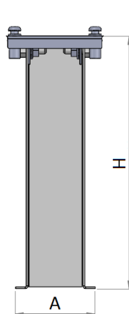
Podstawa do wbetonowania
