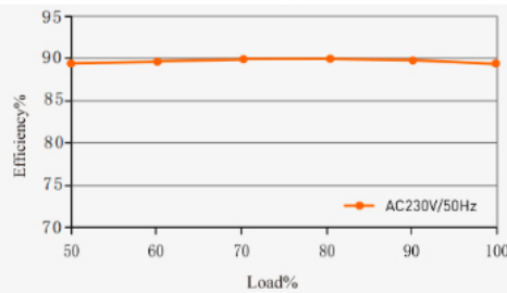
wydajność vs obciążenie / efficiency vs load
