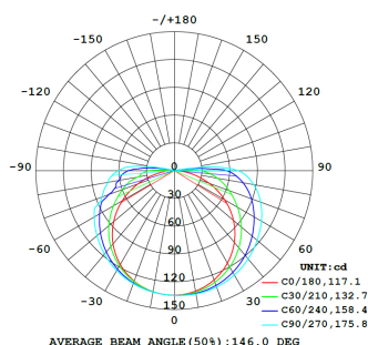
Wykres rozsyłu światłości: Luminous intensity distribution diagram
