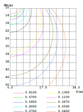
Wartość natężenia oświetlenia w zależności od wysokości montażu: Co plane ISOLUX diagram (unit:lx)
