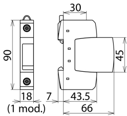
Rysunek wymiarowy DG S 600
