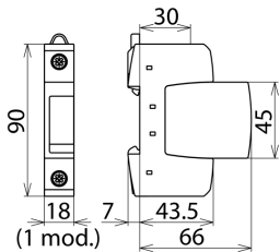
Rysunek wymiarowy DG S 75
