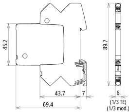
Rysunek wymiarowy BCO ML2 BPD 24
