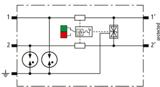
Schemat połączeń BCO ML2 BE HF 5
