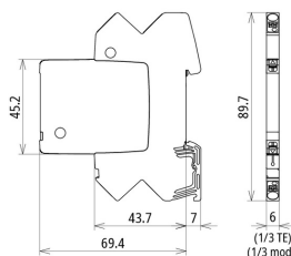
Rysunek wymiarowy BCO ML2 BD 12
