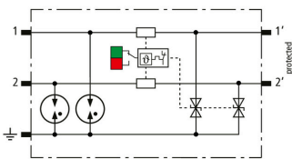
Schemat połączeń BCO ML2 BE 48
