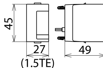
Rysunek wymiarowy DG MOD E DC 900
