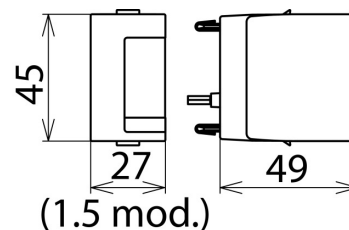
Rysunek wymiarowy DG MOD E DC 60
