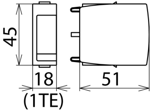
Rysunek wymiarowy DG MOD H PV 750
