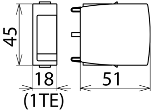
Rysunek wymiarowy DG MOD H PV 600
