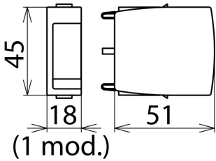
Rysunek wymiarowy DGP C MOD
