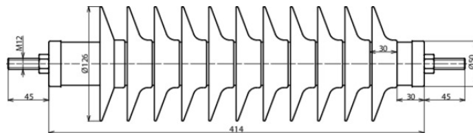
Rysunek wymiarowy DMI 45 10 1 H
