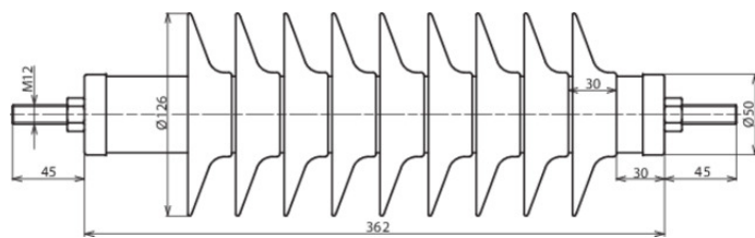
Rysunek wymiarowy DMI 36 10 1 H
