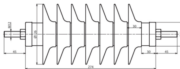
Rysunek wymiarowy DMI 33 10 1 H
