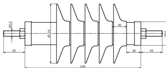
Rysunek wymiarowy DMI 27 10 1 H
