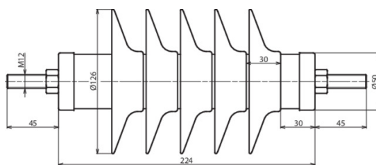
Rysunek wymiarowy DMI 24 10 1 H
