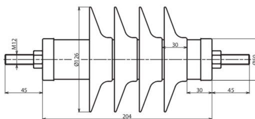
Rysunek wymiarowy DMI 21 10 1 H
