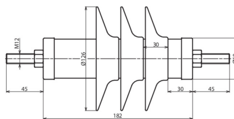
Rysunek wymiarowy DMI 18 10 1 H
