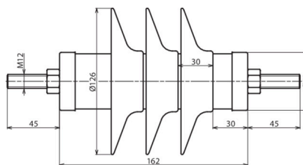
Rysunek wymiarowy DMI 15 10 1 H
