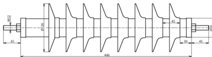
Rysunek wymiarowy DMI 48 10 1 N
