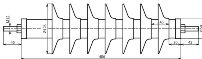
Rysunek wymiarowy DMI 42 10 1 N
