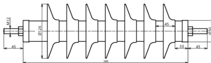
Rysunek wymiarowy DMI 39 10 1 N
