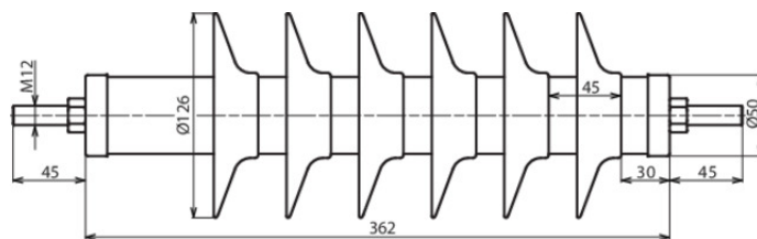
Rysunek wymiarowy DMI 36 10 1 N
