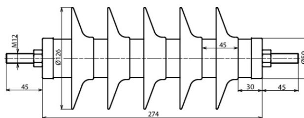
Rysunek wymiarowy DMI 33 10 1 N
