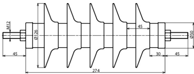
Rysunek wymiarowy DMI 31 10 1 N
