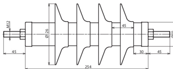
Rysunek wymiarowy DMI 30 10 1 N
