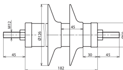
Rysunek wymiarowy DMI 18 10 1 N
