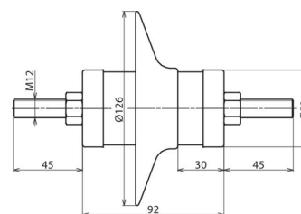
Rysunek wymiarowy DMI 3 10 1 N
