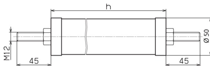
Rysunek wymiarowy DMI 24 10 1 L
