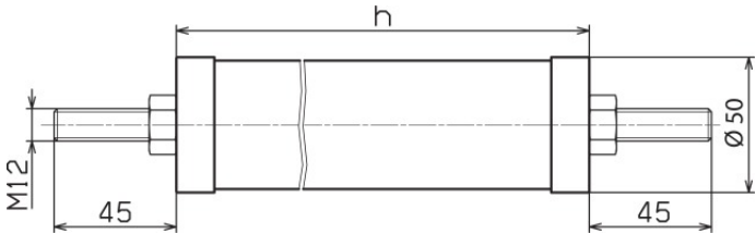
Rysunek wymiarowy DMI 18 10 1 L
