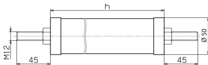
Rysunek wymiarowy DMI 3 10 1 L
