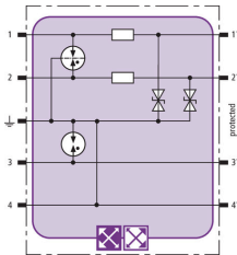
Schemat połączeń BXT ML2 BE S 5
