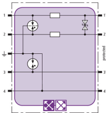
Schemat połączeń BXT ML2 BD S 5
