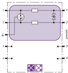
Schemat połączeń BXT ML2 BD 180
