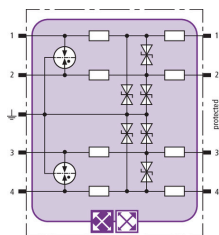
Schemat połączeń BXT ML4 BE C 24
