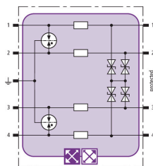
Schemat połączeń BXT ML4 BC 24
