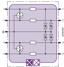
Schemat połączeń BXT ML4 BE 180
