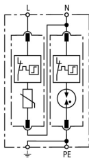
Schemat połączeń DG M TT 2P 320
