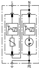
Schemat połączeń DG M TT 2P 275
