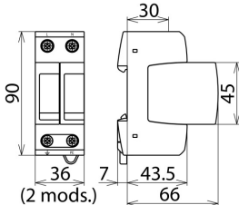
Rysunek wymiarowy DG M TT 2P 275
