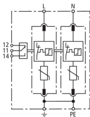
Schemat połączeń DG M TN 275 FM
