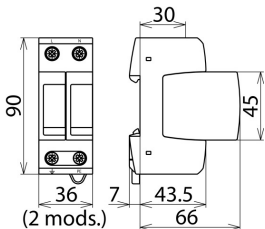
Rysunek wymiarowy DG M TN 275
