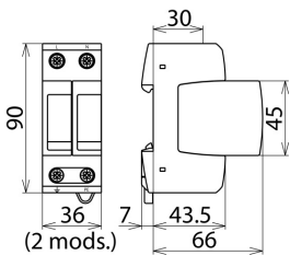
Rysunek wymiarowy DG M TN 150
