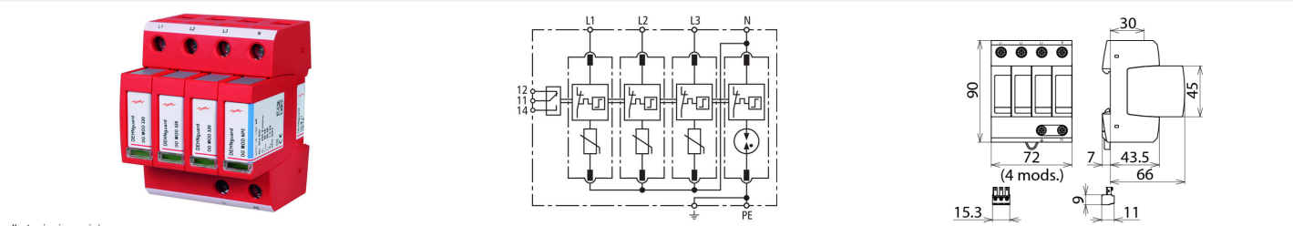
Ilustracje nie są wiążące Schemat połączeń DG M TT 320 FM Rysunek wymiarowy DG M TT 320 FM
