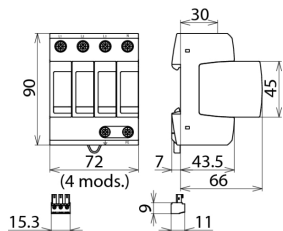
Rysunek wymiarowy DG M TT 275 FM
