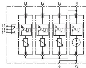
Schemat połączeń DG M TT 275 FM
